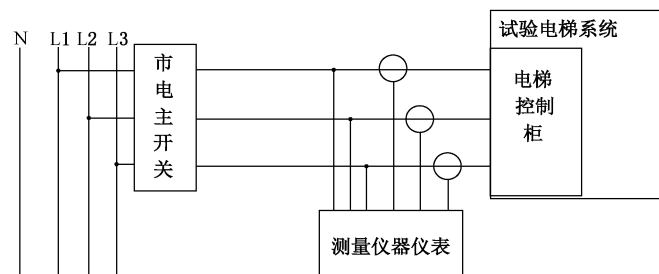
图 2 不配置电源装置的电梯消耗市电电能测量接线示意图
