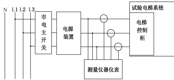
图 1 储能逆变运行时间试验接线示意图
