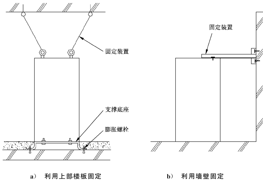
图 5 防止控制柜倾覆或移位措施示例
