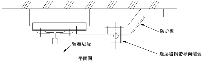
平面图
