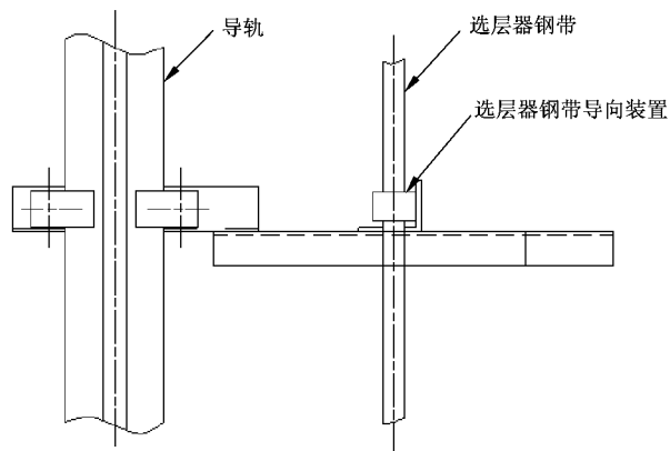
立面图
