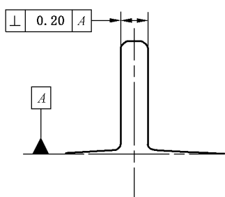
图7 导向面中心线对底部平面的垂直度
