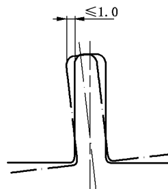
图 4 导向面扭曲度
