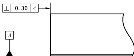
图 5 端面对底平面垂直度
